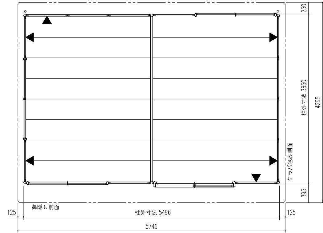
平面図 (S=1/50)
