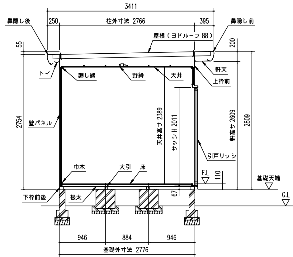
側面断面図 (S=1/50)
