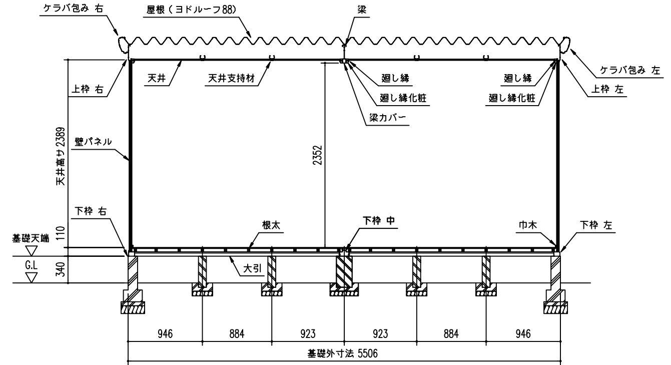
正面断面図 (S=1/50)
