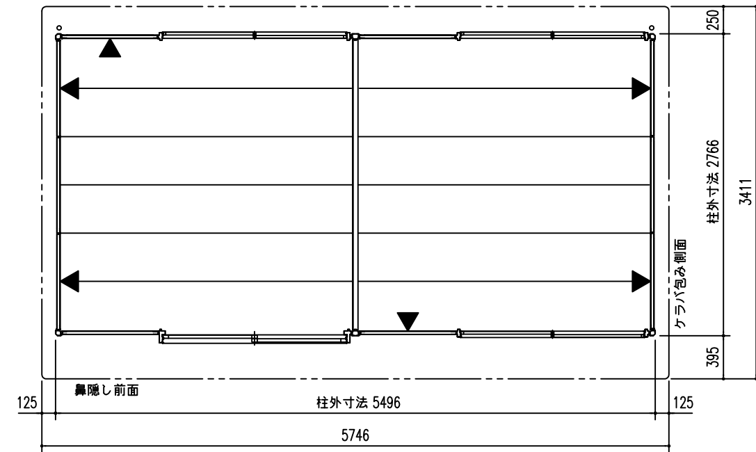
平面図 (S=1/50)
