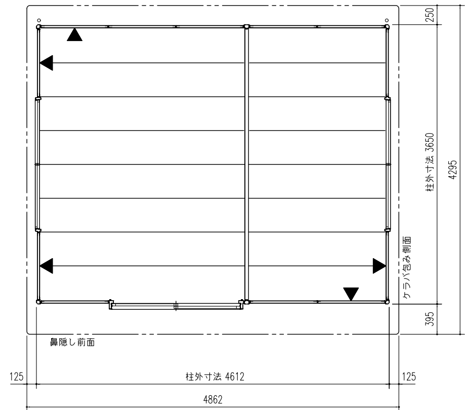
平面図 (S=1/50)
