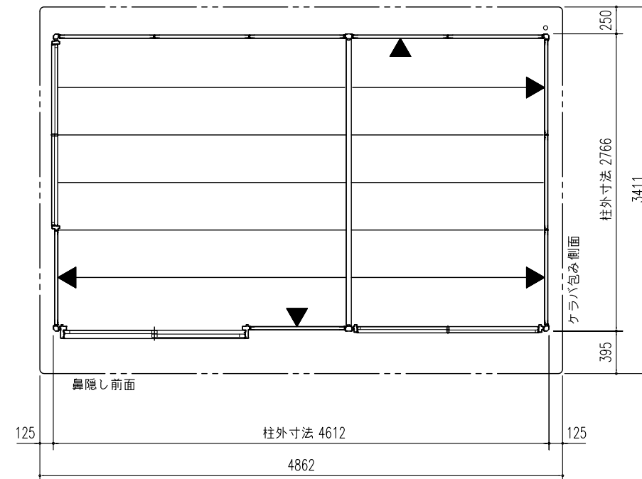
平面図 (S=1/50)
