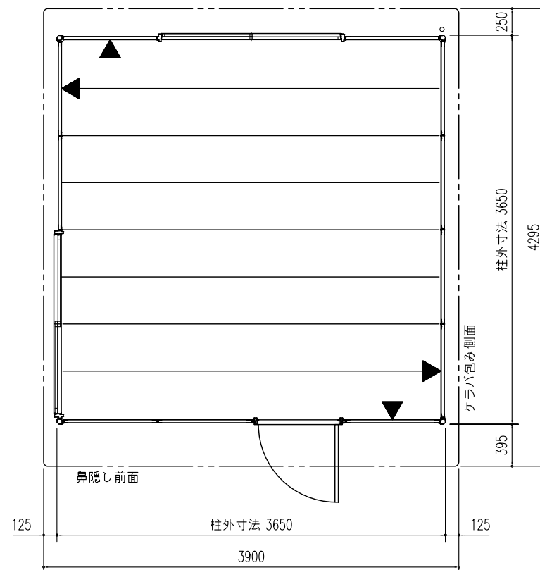
平面図 (S=1/50)
