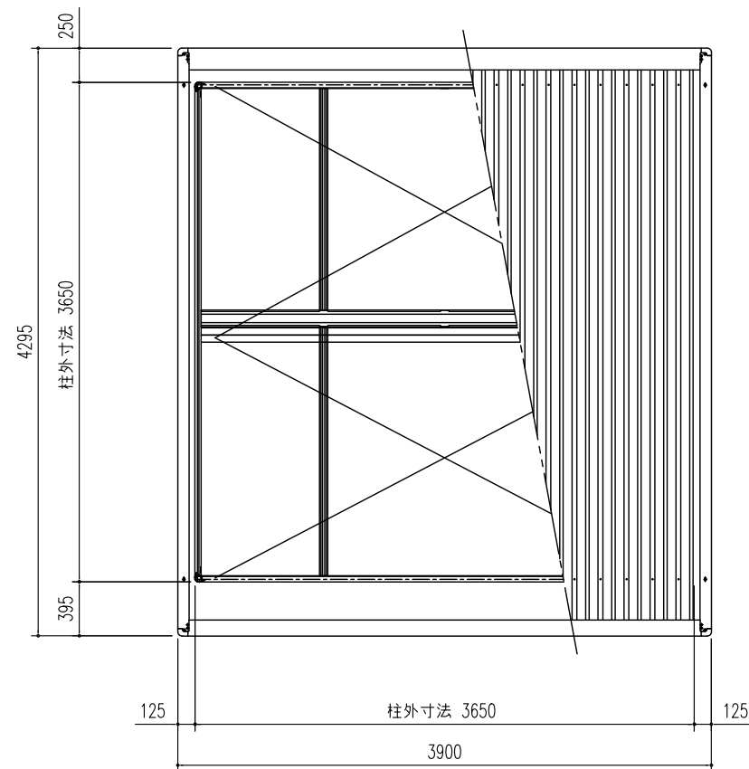
前 小屋伏せ図 (S=1/80)
