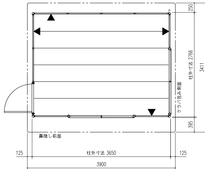
平面図 (S=1/50)
