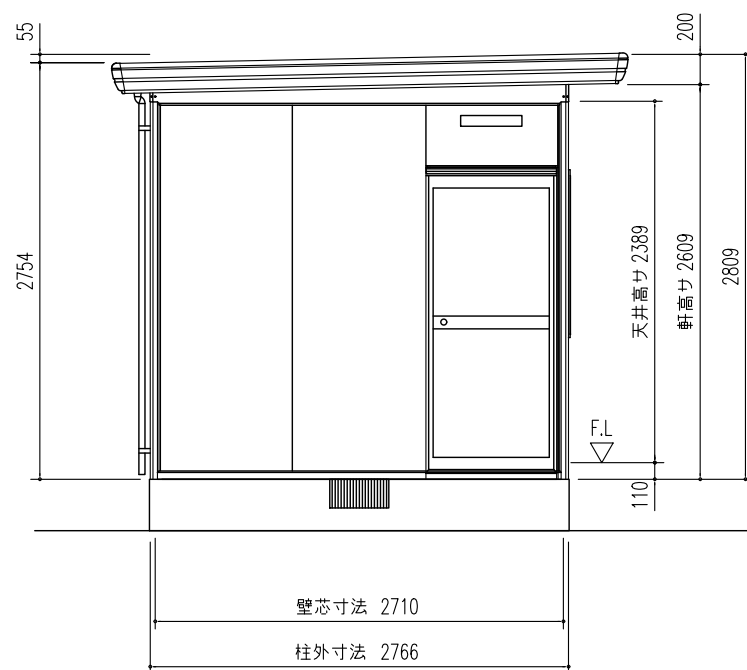
側面立面図 (S=1/50)
