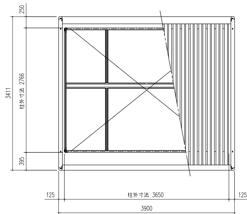
前 小屋伏せ図 (S=1/80)
