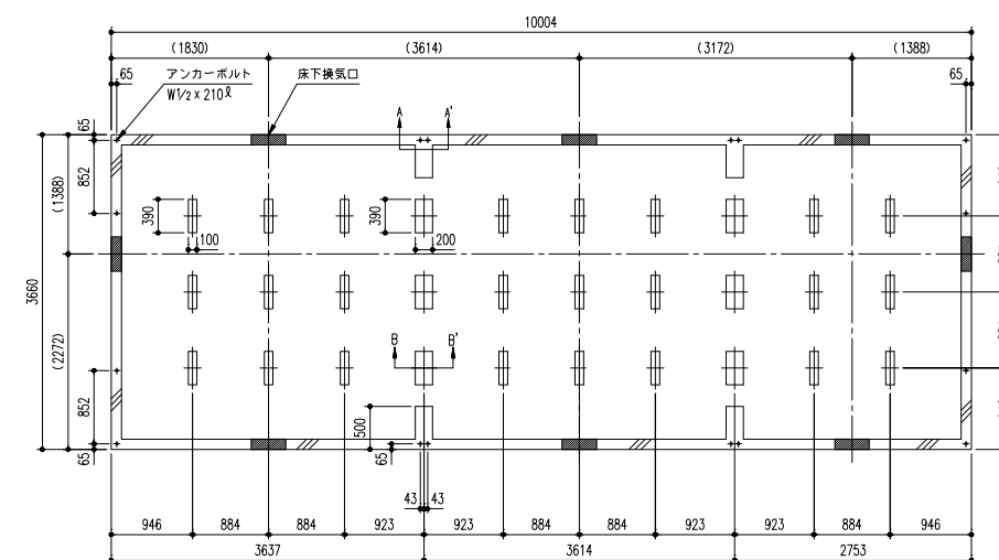
YHF-5520型(22疊)
