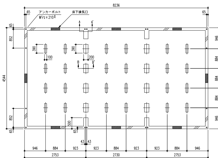
YHF-4525型(22.5畳)
