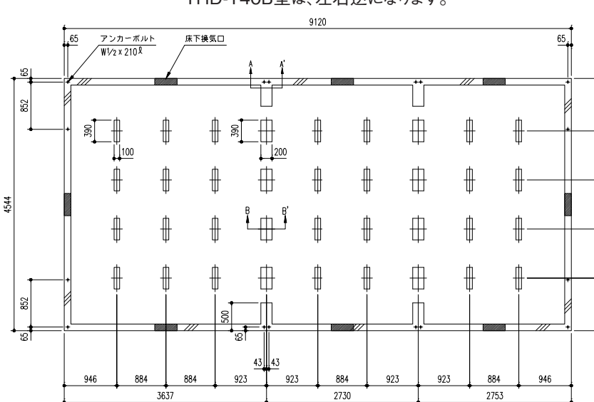
YHF-5025型(25疊)
