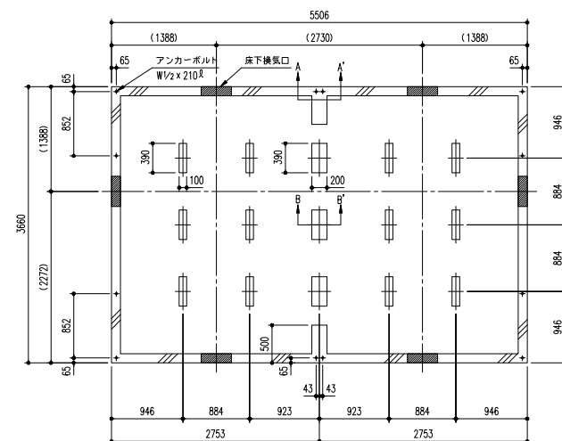
YHF-3025型(15畳)
