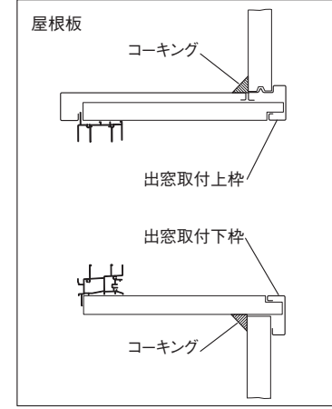
サッシ形状
