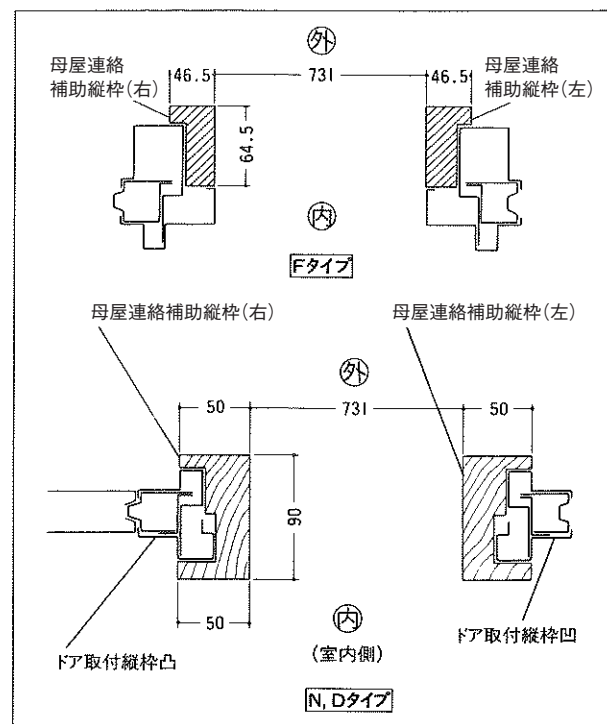
図O-2 横断面図
