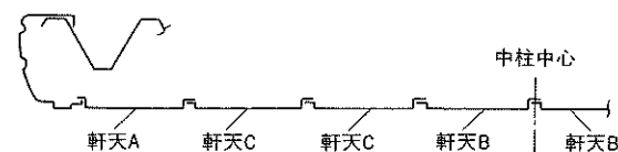
図F27-8 軒天配置図
