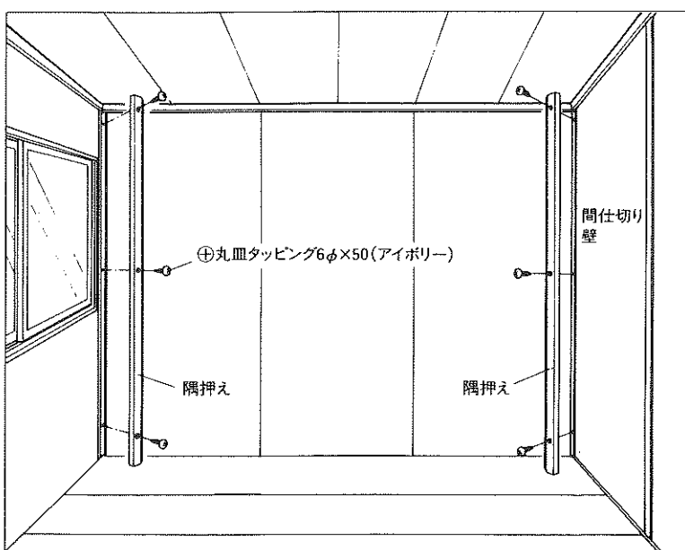
図F26-2 間仕切り付
