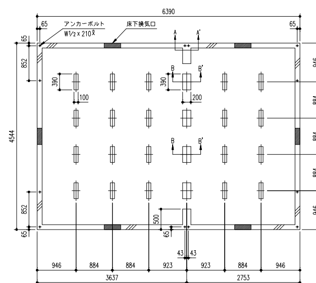
YHF-3525型(17.5畳)
