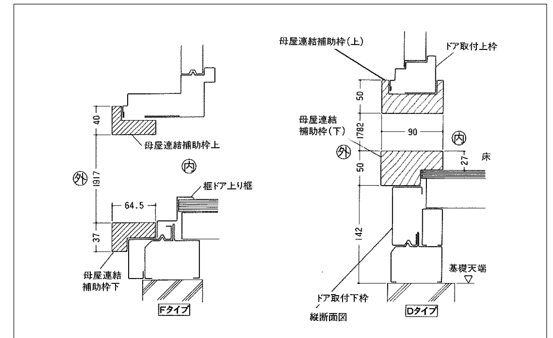
図O-4 縦断面図
