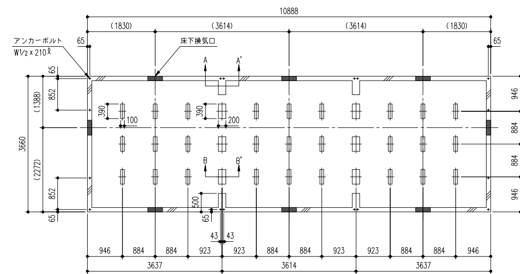
YHF-6025型(30畳)
