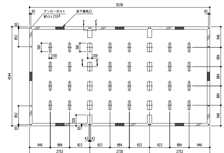
YHF-4025型(20畳)
