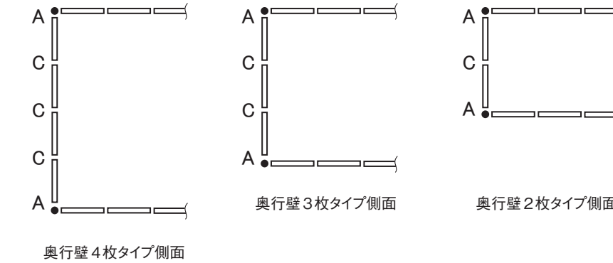
壁取付金具・ブレースドパネル取付金具配置図
