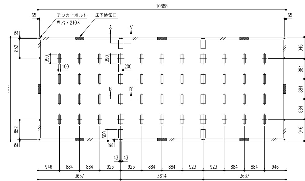
YHF-6025型(30畳)
