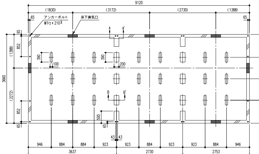
YHF-5025型(25疊)
