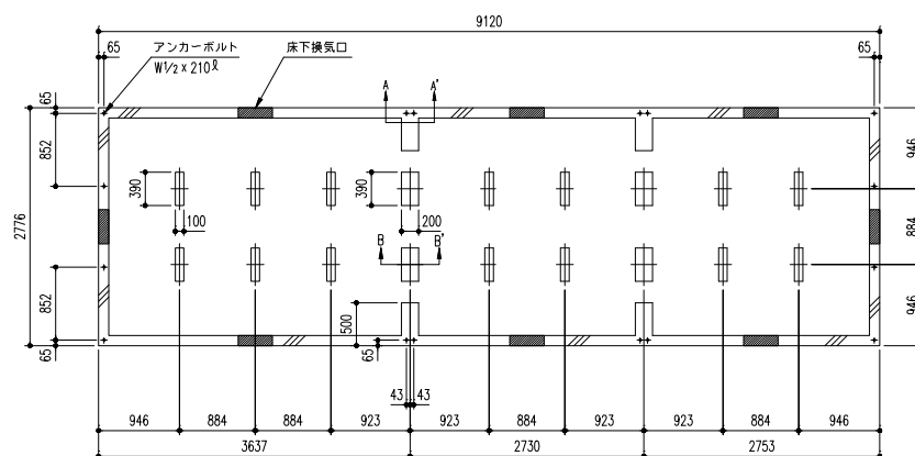
YHF-5015型(15疊)
