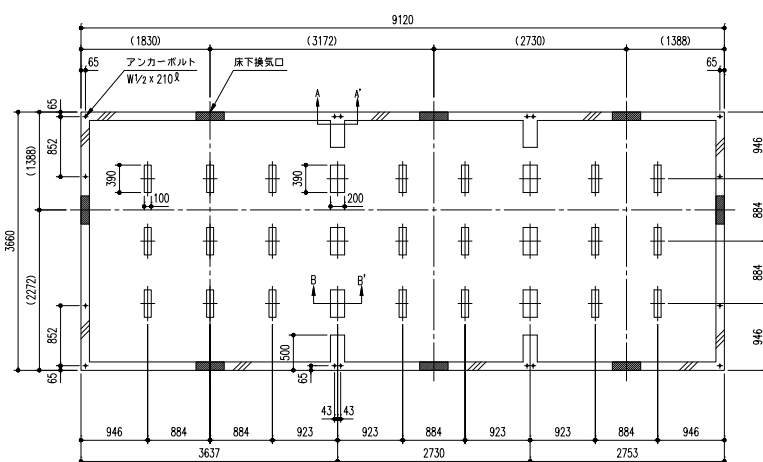
YHF-4525型(22.5畳)
