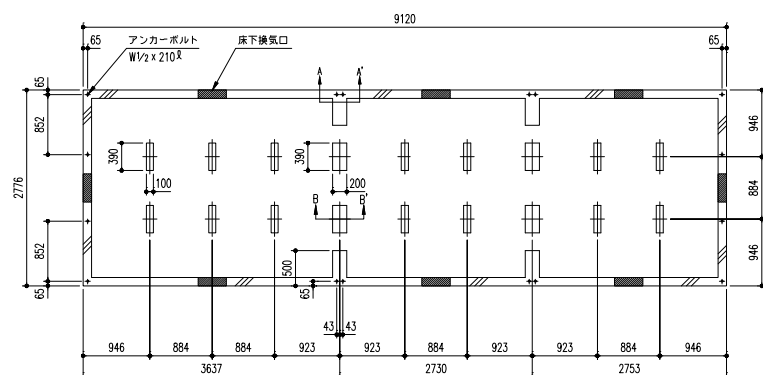
YHF-4515型(13.5疊)
