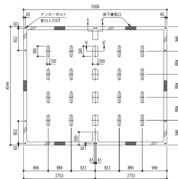
YHF-3025型(15畳)
