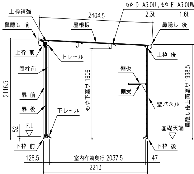
矩計図 (S=1/50)
