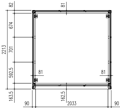
床伏図 (S=1/50)
