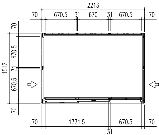
平面図 (S=1/50)
