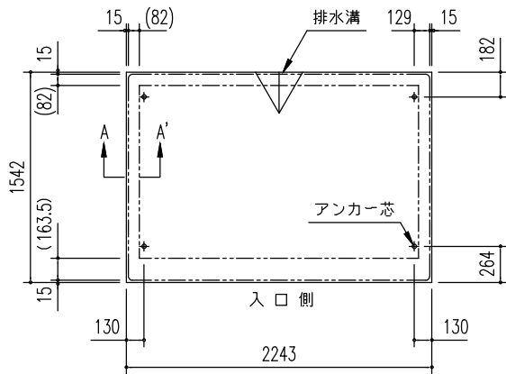
土間基礎伏図 (S=1/50)
