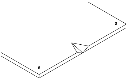
土間基礎排水溝施工例 (注)排水方法は、現場の実状にあわせて設計してください。
