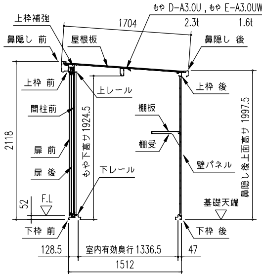
矩計図 (S=1/50)
