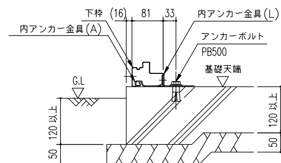
A ~ A' 断面
