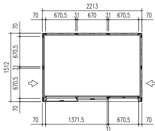
平面图 (S = 1/50)
