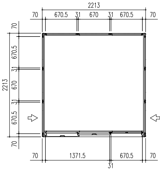
平面図 (S = 1/50)
