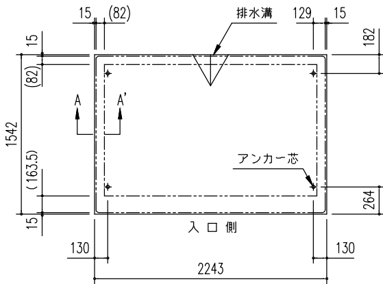
土間基礎伏図 (s=1/50)
