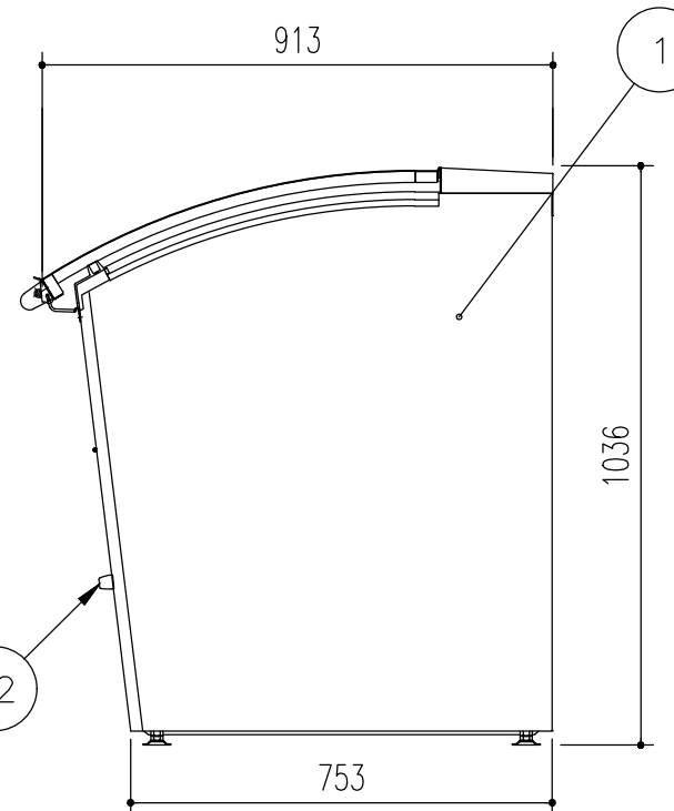
側面立面図
