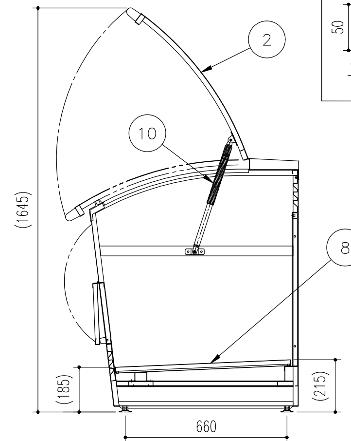
側面立面図
