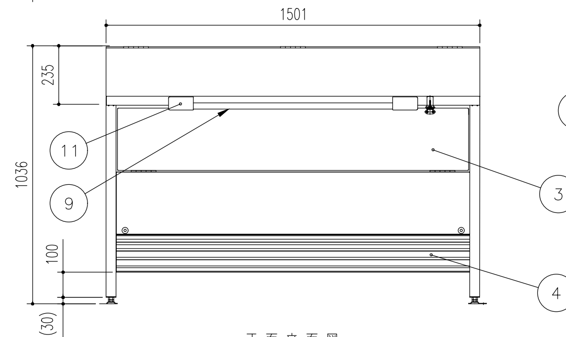
正面立面図
