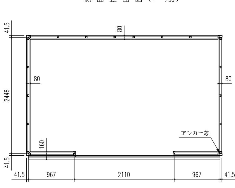
床 伏 図 (S = 1/50)
