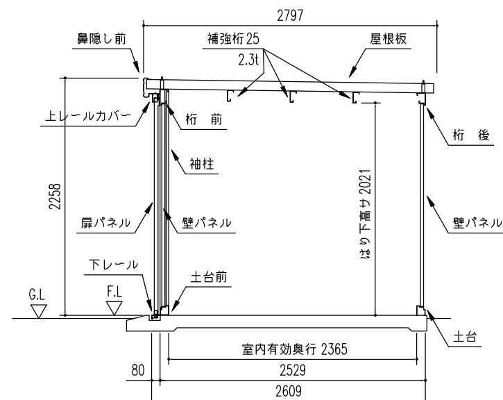
矩 計 図 (S = 1/50)
