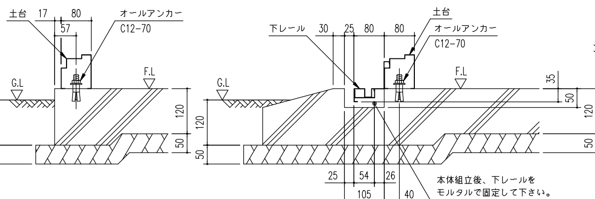
A ~ A' 断面
