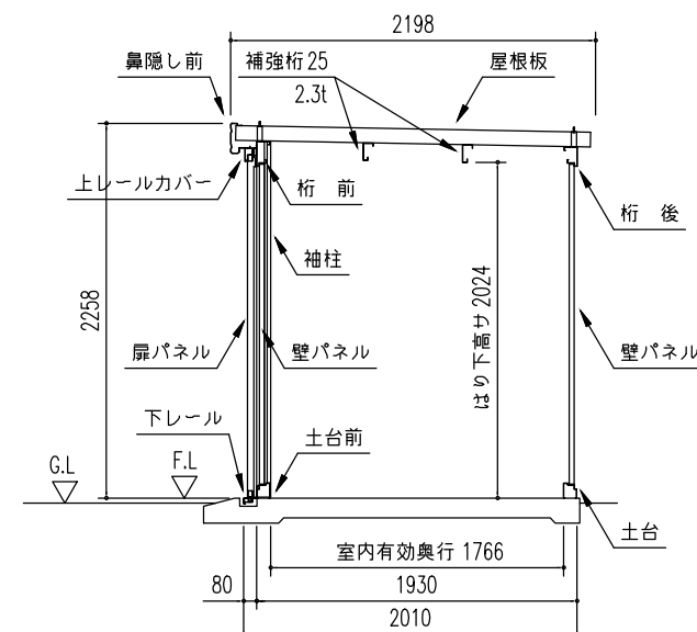
矩 計 図 ( S = 1/50 )
