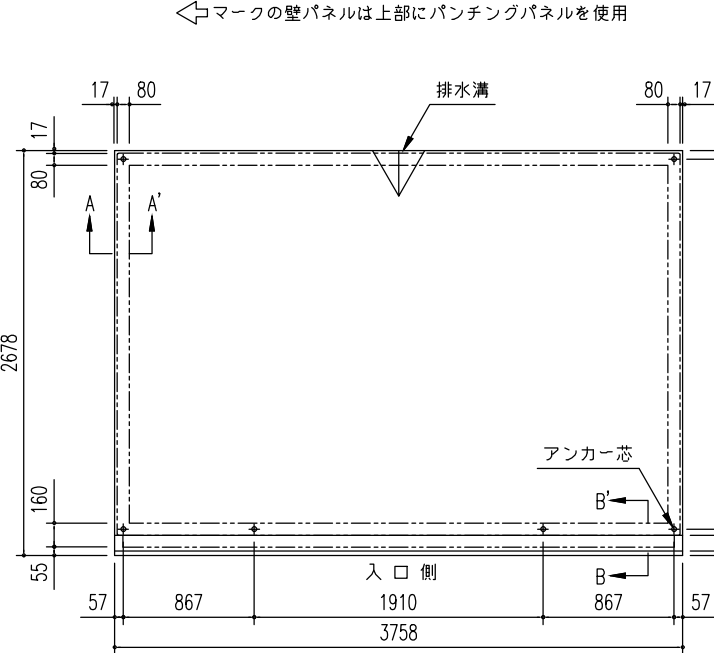
土 間 基 礎 伏 図 (S = 1/50)
