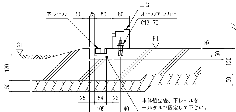
B ~ B' 断 面
