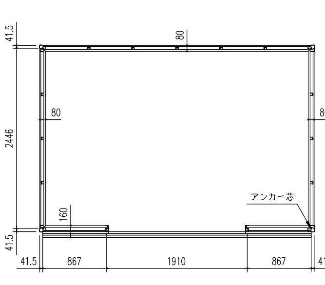
床 伏 図 (S = 1/50)
