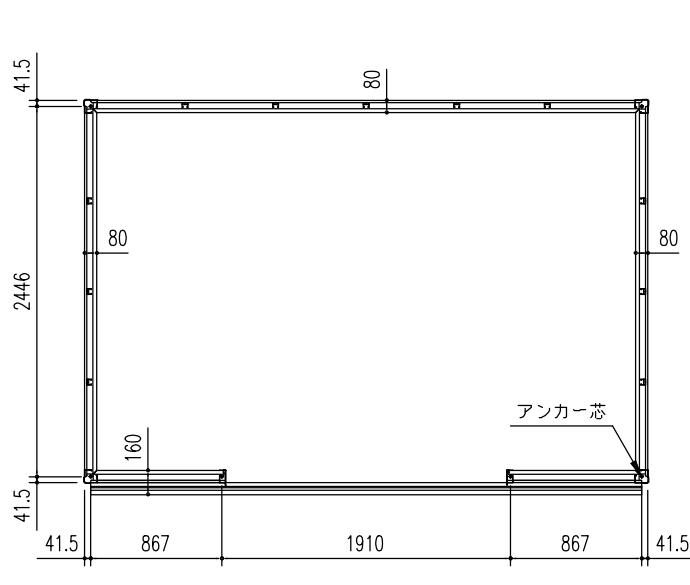
床伏図 (S = 1/50)
