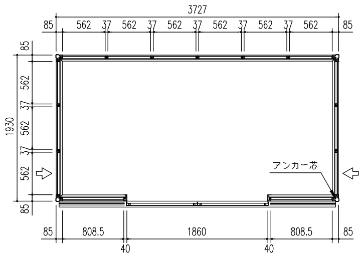
平面図 (S = 1/50)
