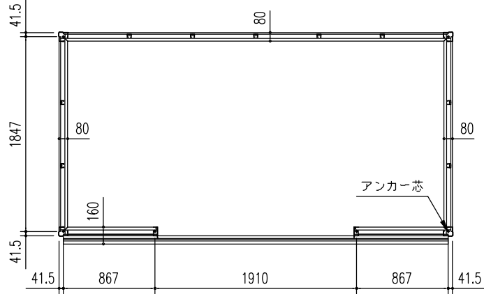
床 伏 図 (S = 1/50)
