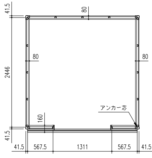
床伏図 (S = 1/50)
