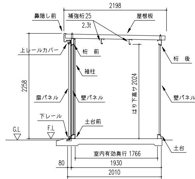
矩計図 (S = 1/50)
