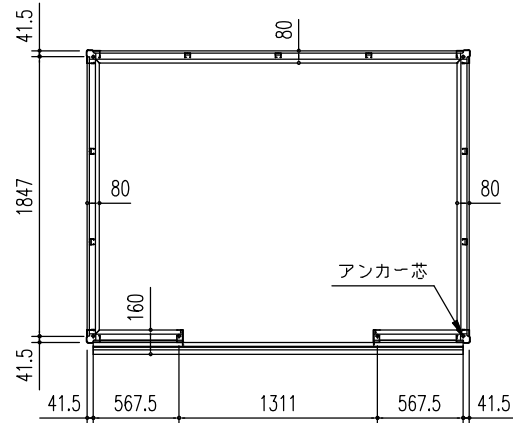
床 伏 図 (S = 1/50)
