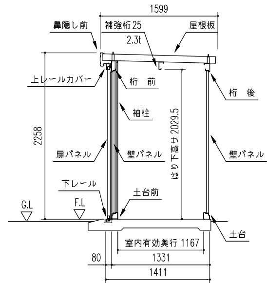
矩計図 (S = 1/50)
