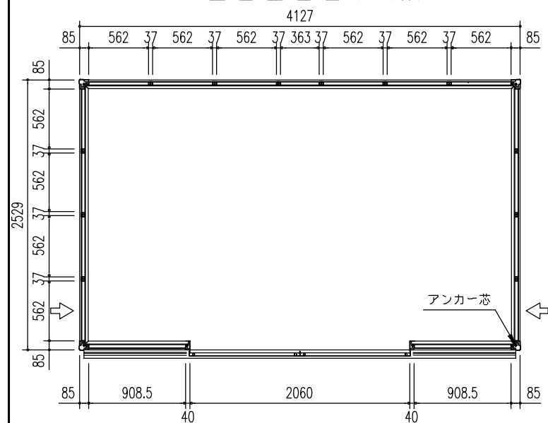
平面図 (S = 1/50)
