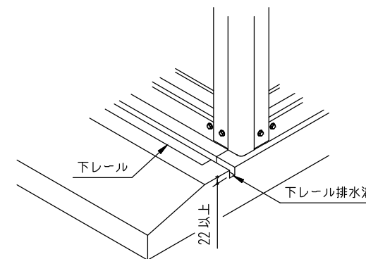
下レベル排水施行例
