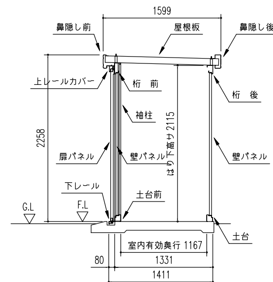
矩 計 図 (S = 1/50)
