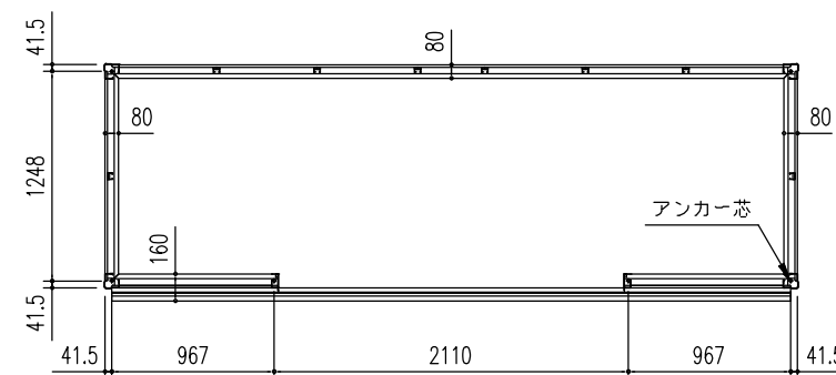
床 伏 図 (S = 1/50)
