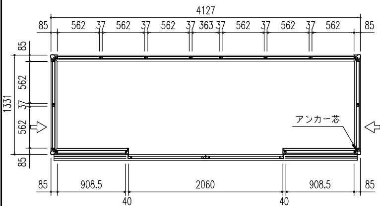
平面図 (S=1/50)
