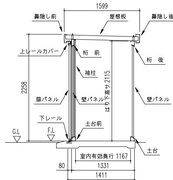
矩計図 (S=1/50)
