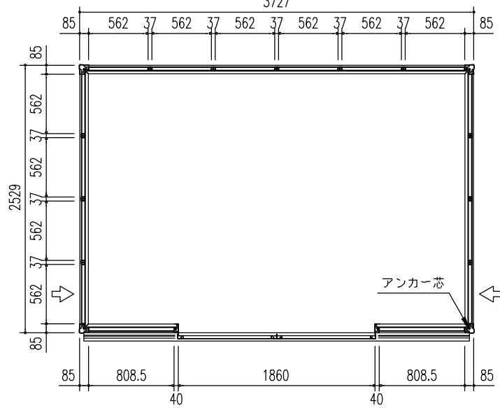
平面図 (S = 1/50)
