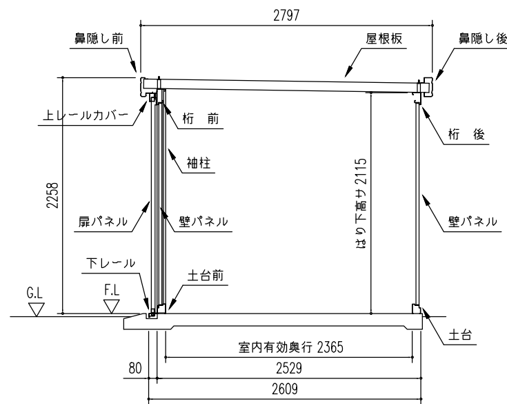
矩計図 (S = 1/50)
