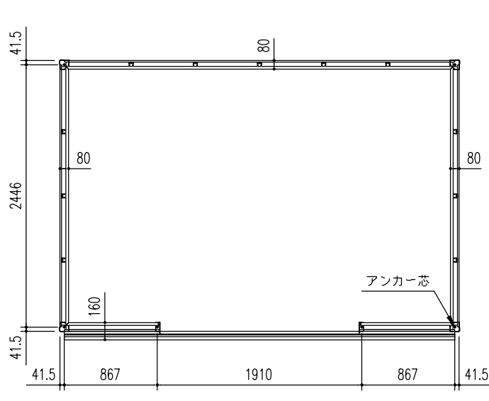
床伏図 (S=1/50)
