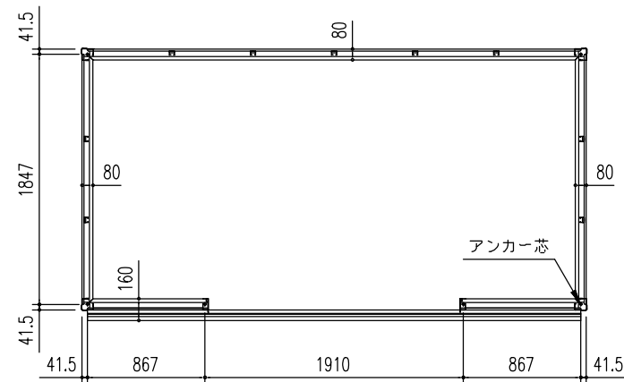
床 伏 図 (S = 1/50)
