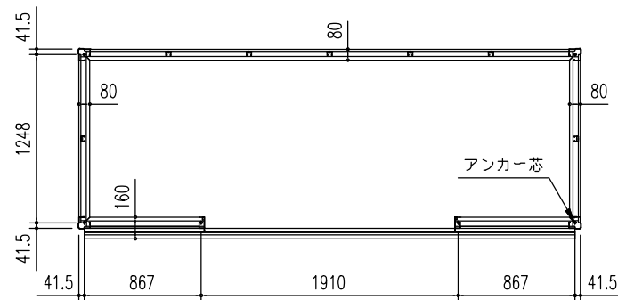
床 伏 図 (S = 1/50)
