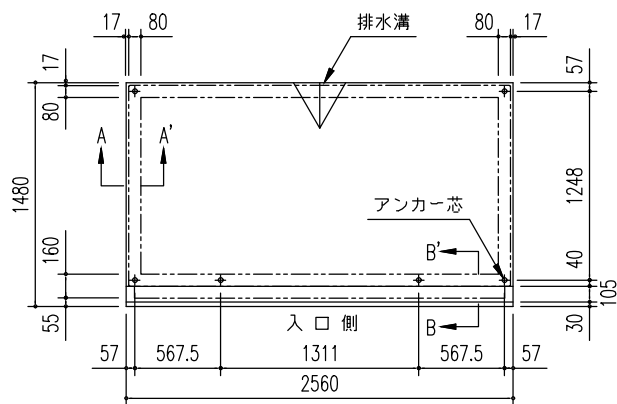
土 間 基 礎 伏 図 (S = 1/50)
