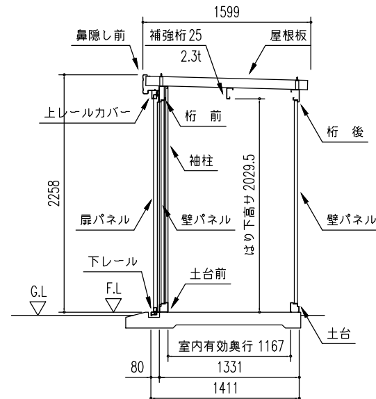
矩計図 (S = 1/50)
