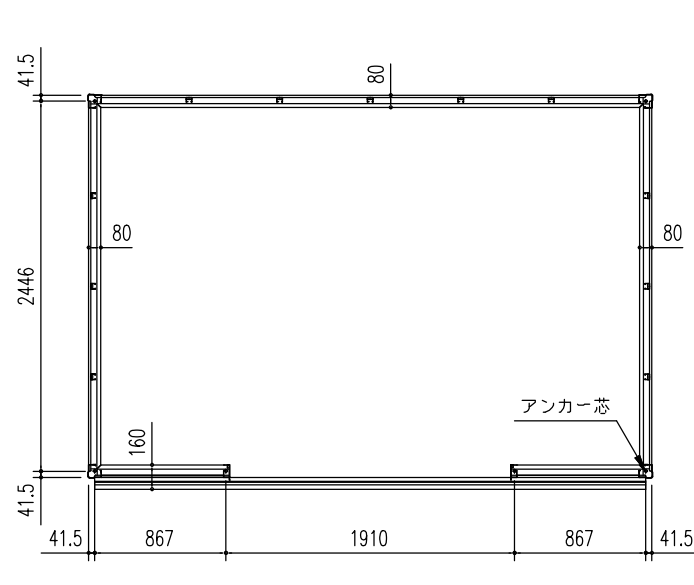
床伏図 (S = 1/50)
