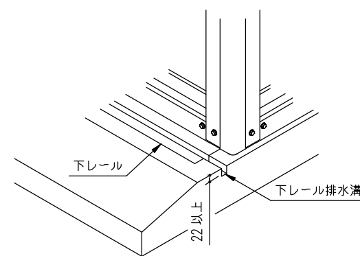
下レール排水施工例
