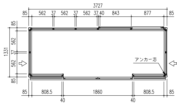
平面図 (S=1/50)
