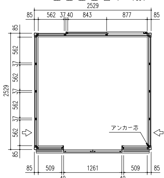
平面図 (S = 1/50)
