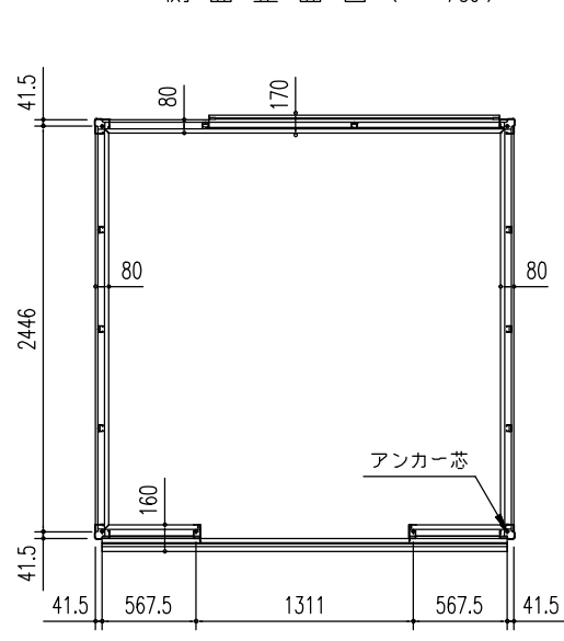
床 伏 図 (S = 1/50)
