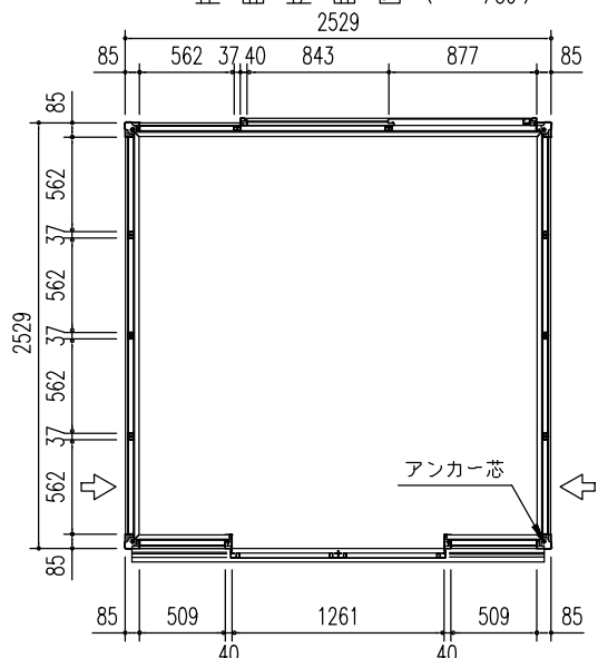
平面図 (S = 1/50)
