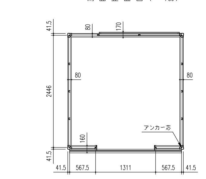
床 伏 図 (S = 1/50)
