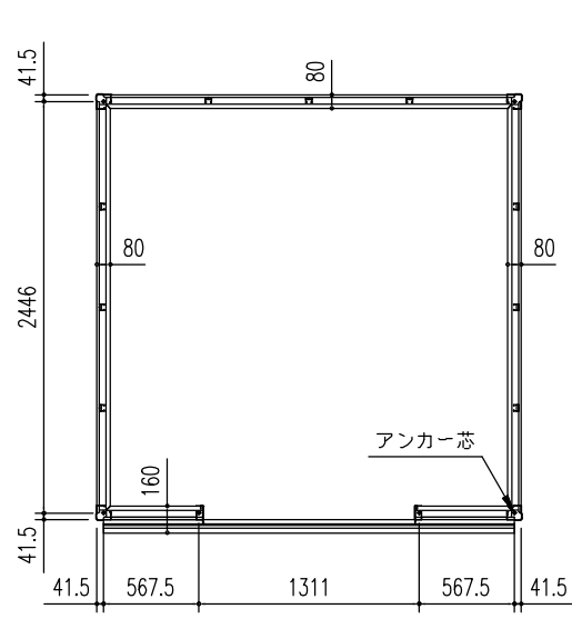
床 伏 図 (S = 1/50)
