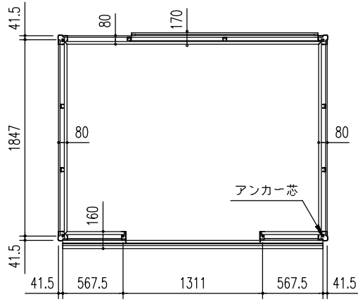
床 伏 図 (S = 1/50)
