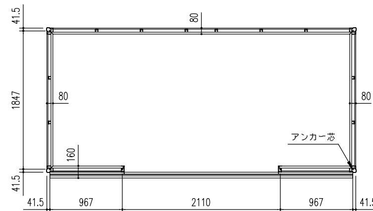
床 伏 図 (S = 1/50)
