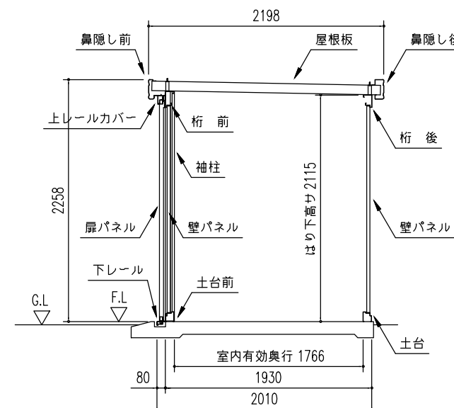
矩 計 図 ( S = 1/50 )
