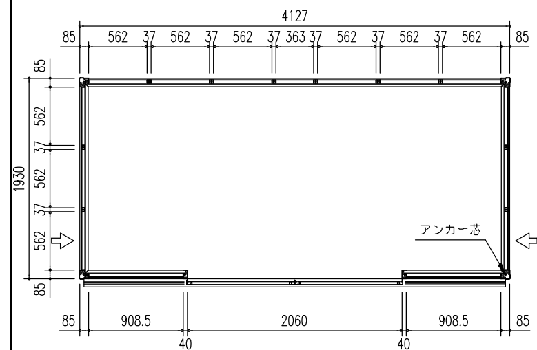
平面図 (S = 1/50)
