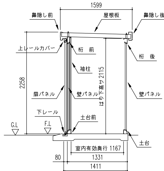
矩計図 (S = 1/50)
