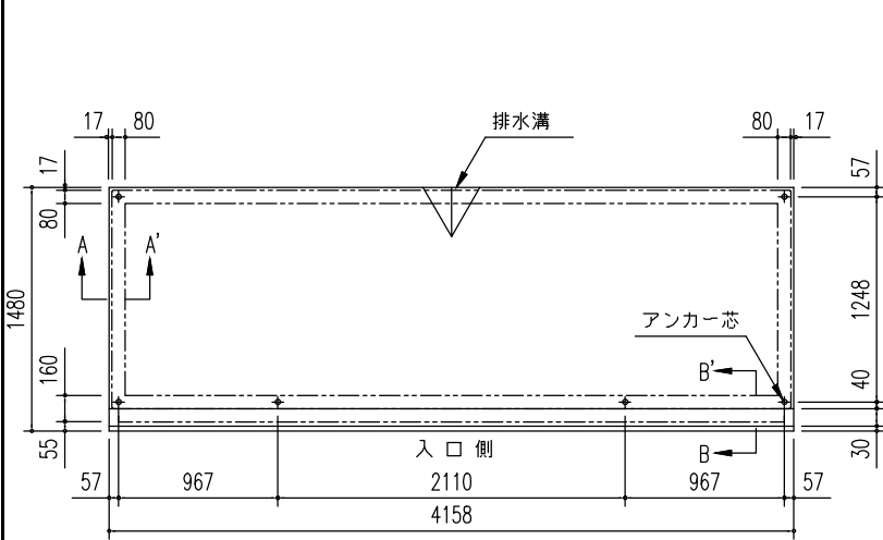
土間基礎伏図 (S = 1/50)
