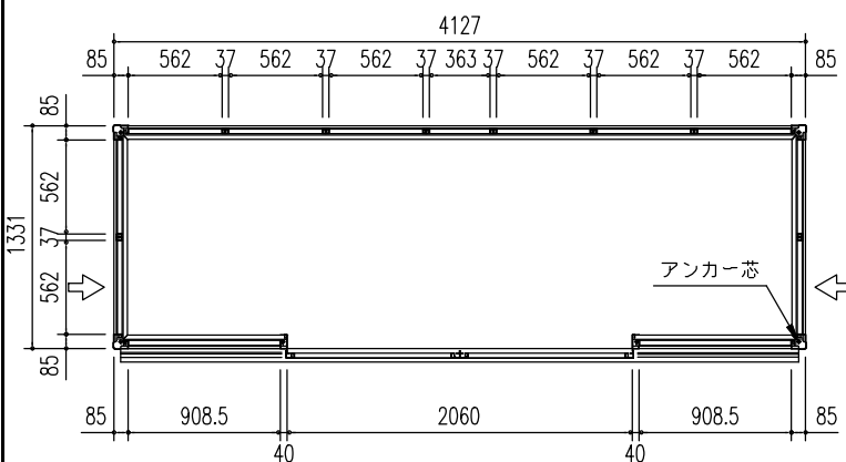
平面図 (S = 1/50)
