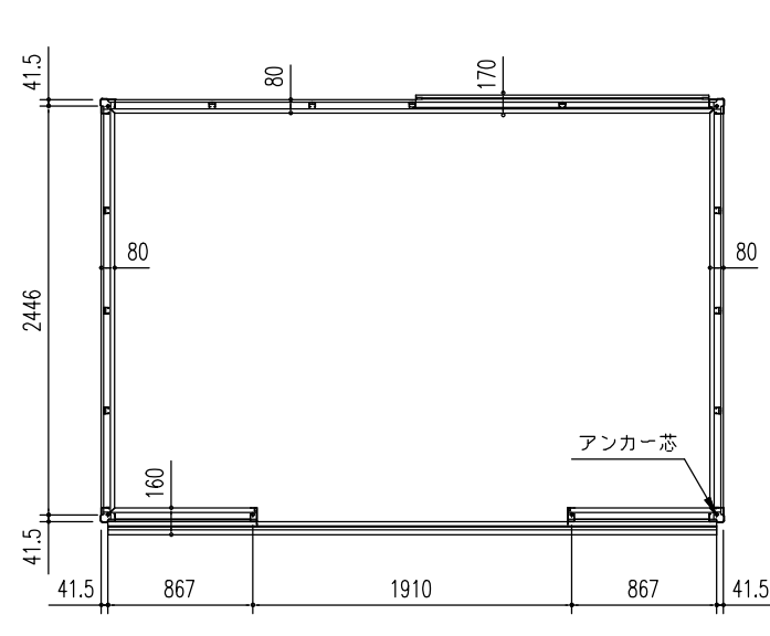
床伏図 (S = 1/50)
