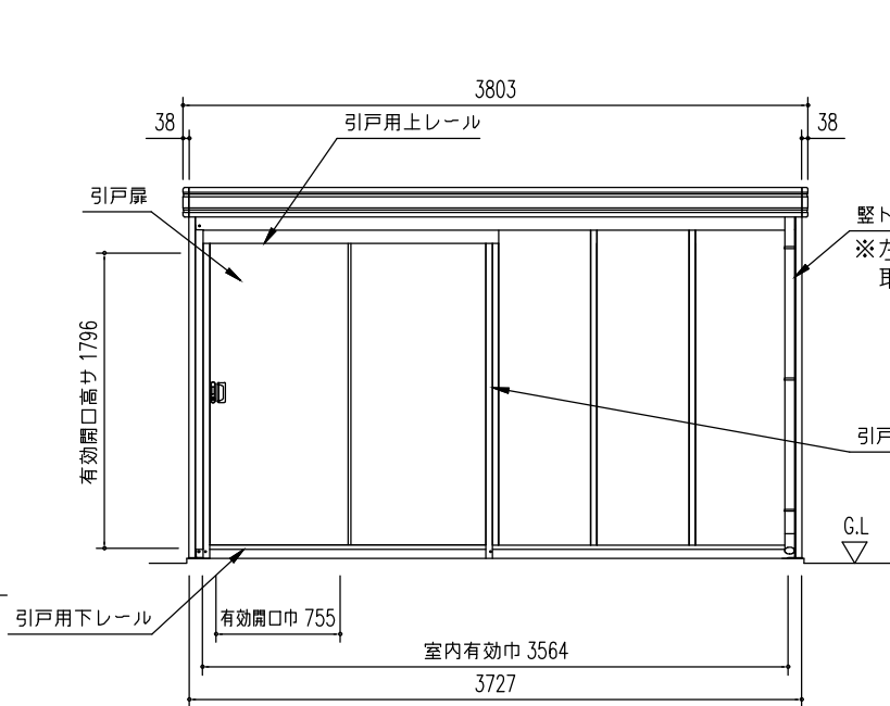
後面立面図 (S = 1/50)
