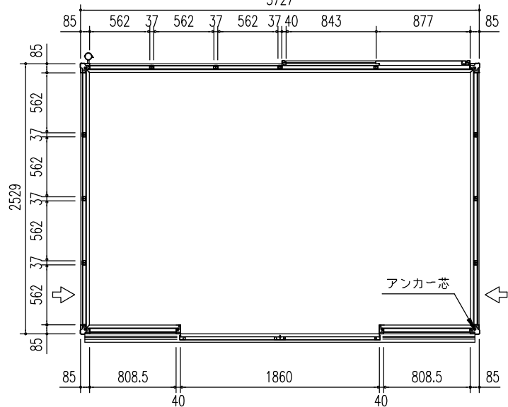
平面図 (S = 1/50)
