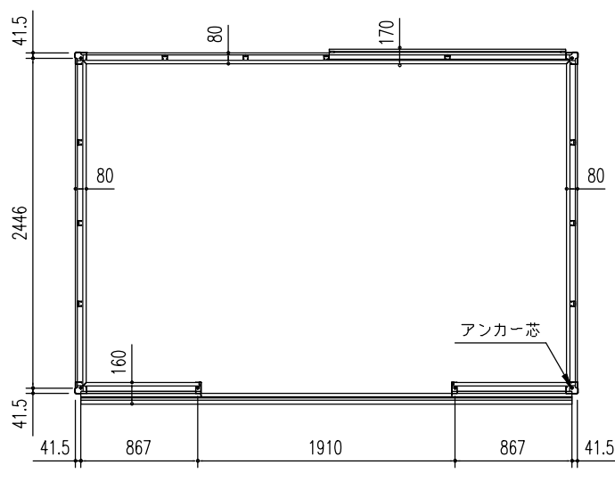
床 伏 図 (S = 1/50)
