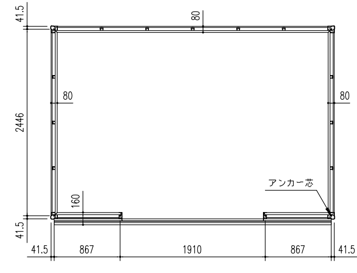
床 伏 図 (S = 1/50)
