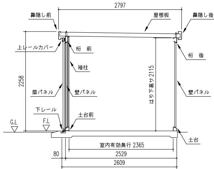
矩計図 (S = 1/50)
