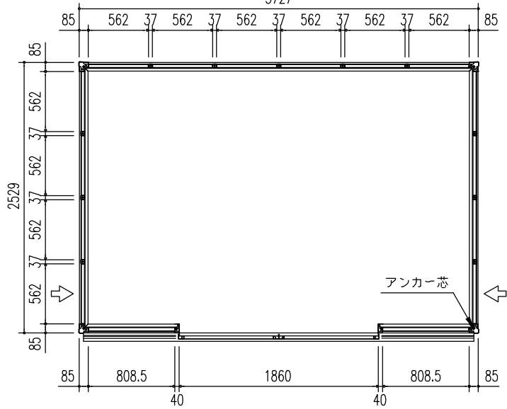
平面図 (S = 1/50)
