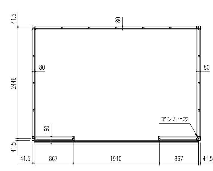
床伏図 (S=1/50)
