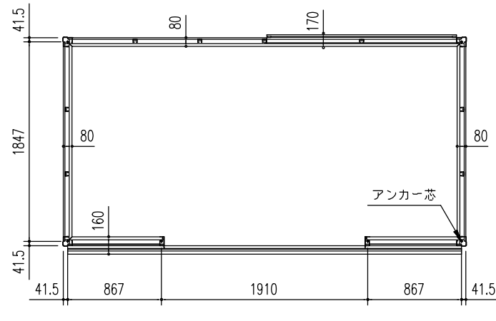
床伏図 (S=1/50)
