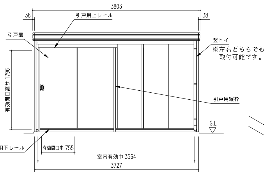
後面立面図 (S=1/50)
