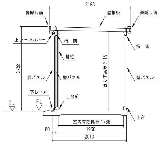
矩計図 (S = 1/50)
