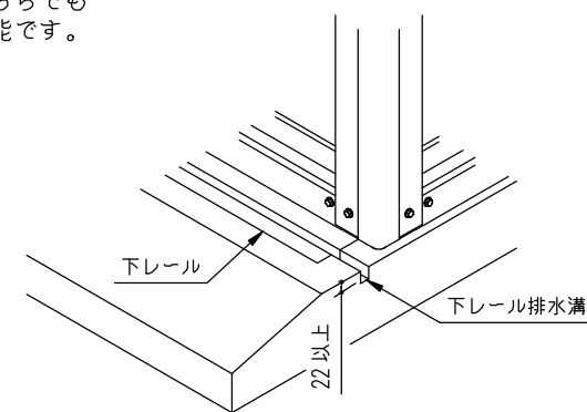
下レール排水施工例
