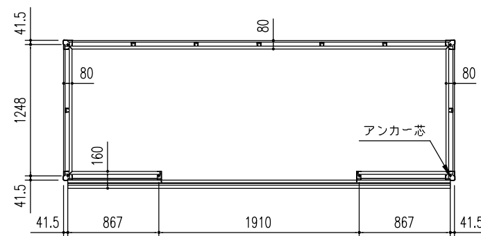
床 伏 図 (S = 1/50)
