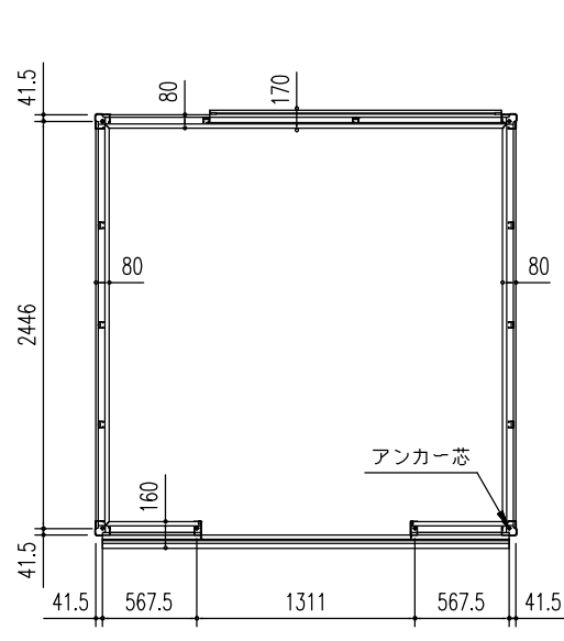
床 伏 図 (S = 1/50)
