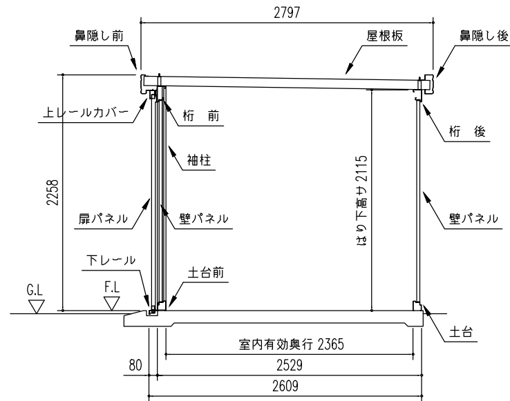
矩計図 (S = 1/50)
