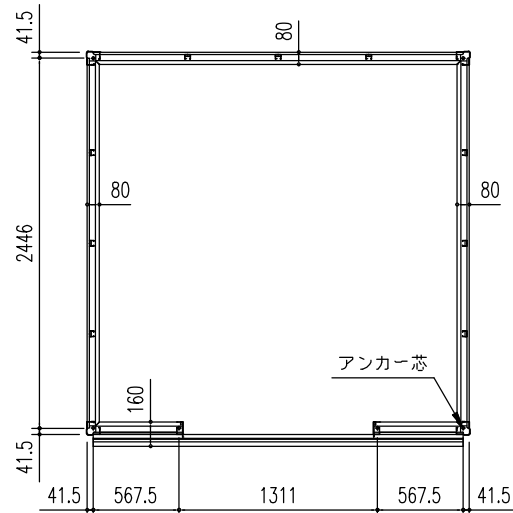
床 伏 図 (S = 1/50)
